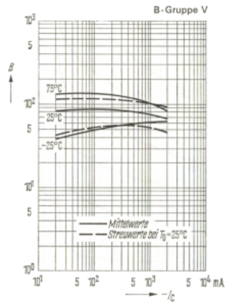
Stromverstärkung B = f(I_C) -U_{CE} = 1 V; T_G = \text{Parameter}
